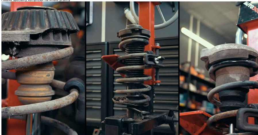
13 Odstráňte horné uloženie vzpery, aby ste sa dostali k protiprachovej manžete a dorazu pružiny
