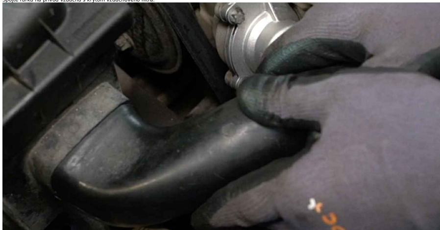
32 Pripevnite sponu na nasávaciu hadičku vzduchového filtra.
