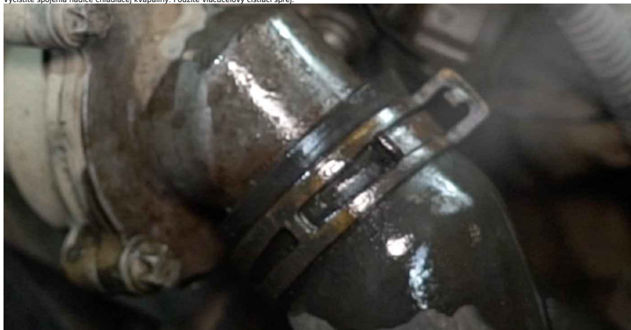
16 Uvoľnite svorky hadičiek chladiacej kvapaliny. Použite hadicové kliešte Clic-R.
