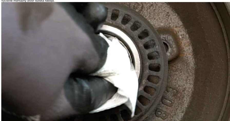
15 Odstráňte vnútornú drážku ložiska kola z brzdového bubna. Použité univerzálny sťahovač.
